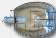
IP 220 G - GRADE, BRAÇO 1 a 2'' E27 / E40 até 250W Medidas 415x 280X130mm
